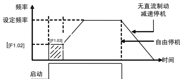
图 6-4 启动与停机频率输出曲线
