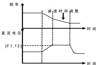
图 6-6 减速中的电压失速保护
