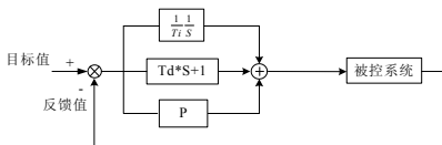
图 6-17 PID 过程示意图
