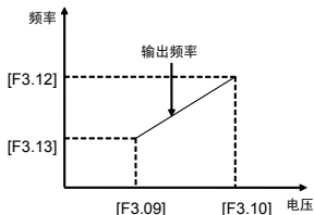
图 6-10 模拟输入量与设定频率对应关系图示
