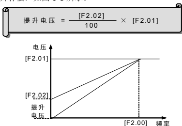
图 6-8 转矩提升示意图
