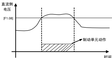
图 6-5 能耗制动
