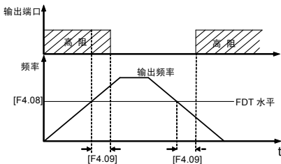
图 6-14 频率水平检测信号 (FDT)
