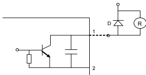
图 6-12 OC 输出端子的内部线路
