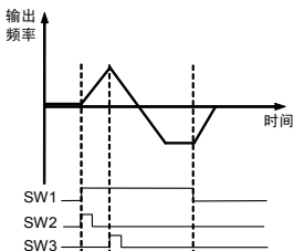
图 6-3 三线控制模式频率输出图
