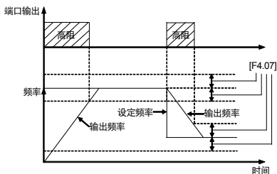
图 6-13 频率到达信号
