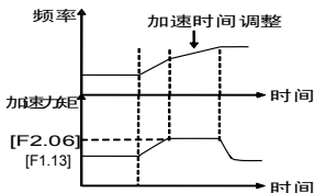
图 6-7 加速力矩与制动力矩示意图
