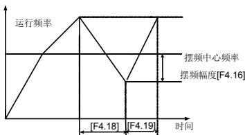
图 6-16 摆频运行过程
