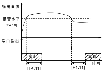
图 6-15 过载报警
