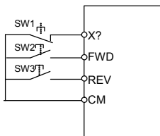
图 6-2 三线控制模式接线图
