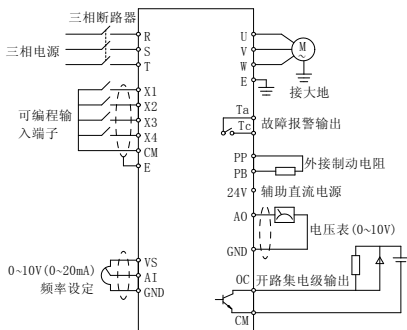
图 3-3 变频器的基本配线
