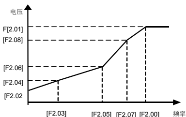
图 6-9 V/F 自定义曲线设定
