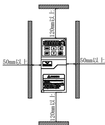
图 2-1-B 安装的间隔距离
