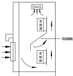
图 2-1-C 多台变频器的安装
