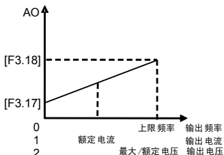
图 6-11 模拟输出端子的模拟输出内容
