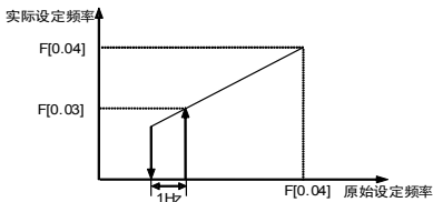
图 6-1 下限频率作用示意图
